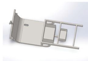
طراحی پیشرفته شاسی و استفاده از پروفیل ۴۰*۵۰ با ضخامت ۲ میلی متر
