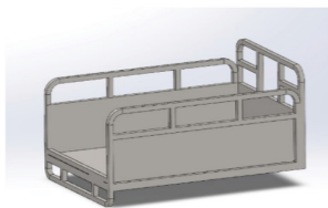
طراحی پیشرفته قسمت بار و استفاده از پروفیل صنعتی ۳۰*۵۰ با ضخامت ۱/۵ میلی متر
